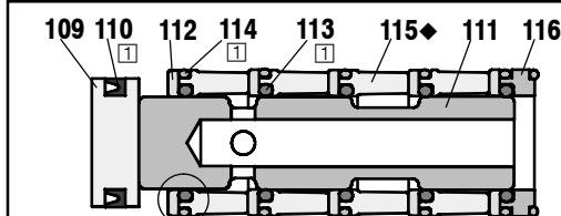
DETALLE DE LA SECCIÓN TRANSVERSAL DE LA VÁLVULA PRINCIPAL DETAIL EN COUPE TRANSVERSALE DE LA SOUPEPE PRINCIPALE
